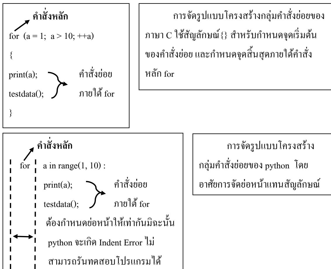
รูปที่ 2.9 แสดงการเปรียบเทียบการจัดรูปแบบโครงสร้างกลุ่มคำสั่งย่อยของภาษา python
