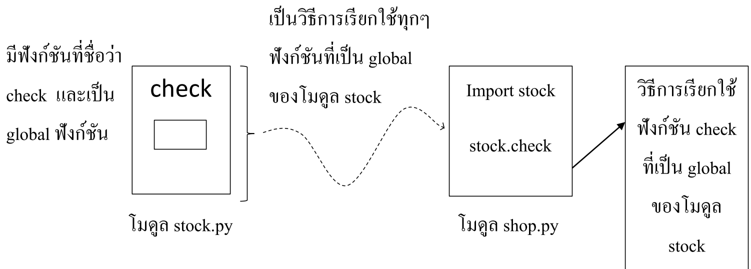
รูปที่ 3 แสดงลักษณะการสร้าง Global ฟังก์ชันและการเรียกใช้งานฟังก์ชันระหว่างโมดูล
