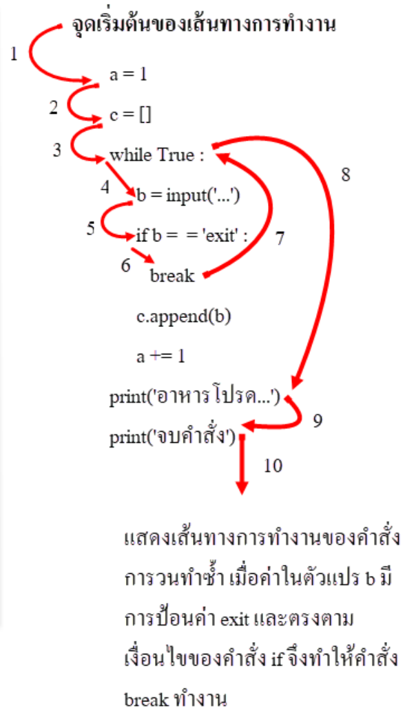
รูปที่ 5.1 แสดงเส้นทางการทำงานของคำสั่งการวนทำซ้ำแบบไม่มีวันสิ้นสุดและวิธีการหยุดการวนทำซ้ำด้วยคำสั่ง break
