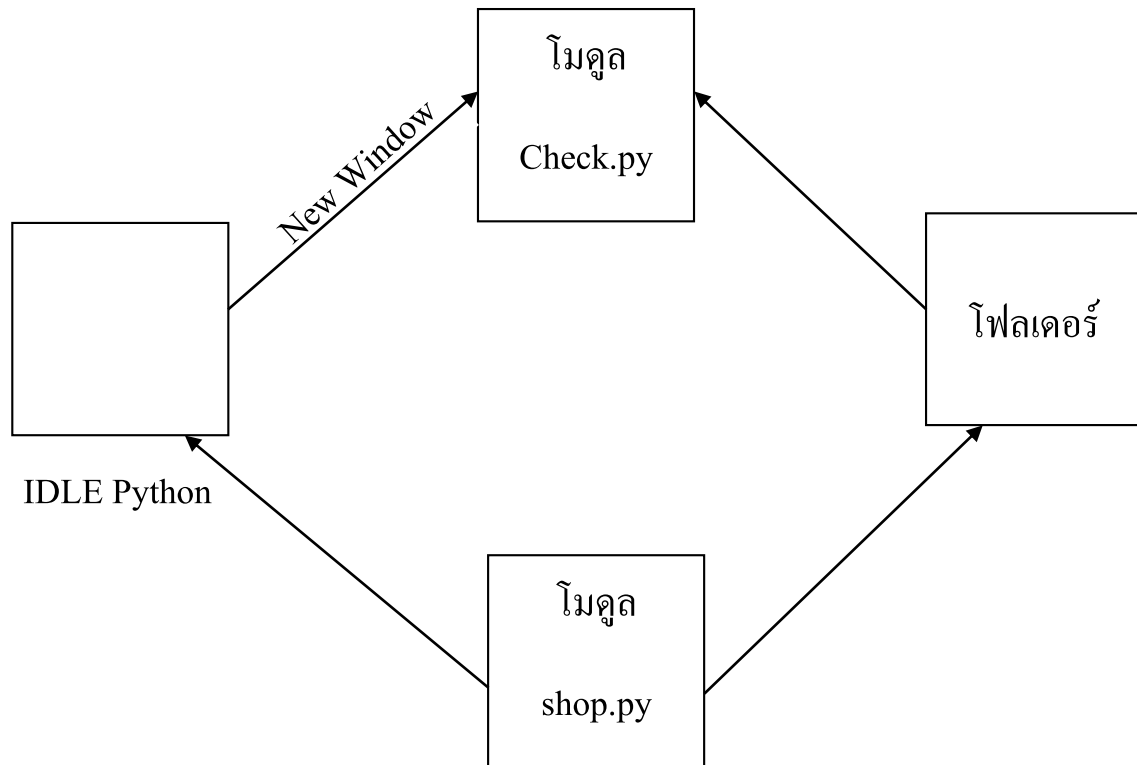
รูปที่ 4 ลำดับการสร้างโมดูลไปเก็บไว้ใน C:\Go Sample
